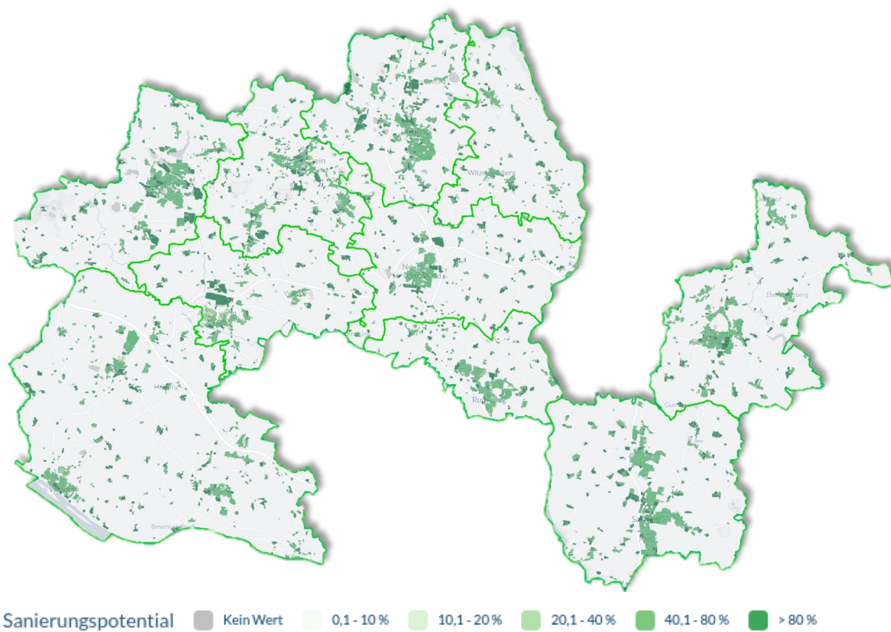
Abbildung 19: Mögliches Sanierungspotenzial
